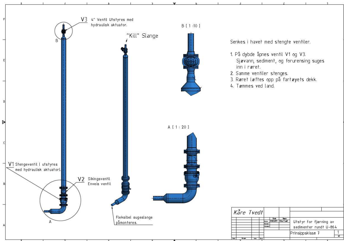
Figur 4-7. Gas-lift teknologi for å suge kvikksølv/masse ved vrak. Prinsippet er basert på differensial trykk ved dybde ved at man blåser røret tomt for vann og slipper ut denne lufta etterpå.
