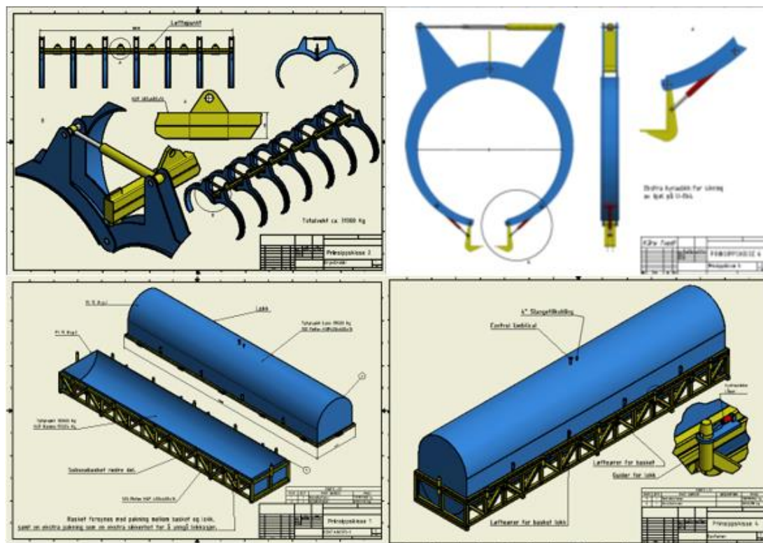
Figur 4-6. Konseptutkast for løfting av vrakdeler mottatt fra Reidar Ulvøy. Konseptet er basert på at man bruker en grabb fra toppen som løfter rundt vrakdeler, disse legges over i en forhåndsplassert lukket container som brukes til å løfte opp vrakdelene til overflate.
