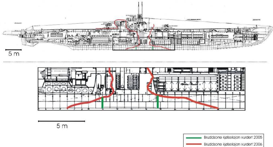
Figur 1-2. Antatt bruddsone for vraket av U-864 som følge av torpedering. Det er stor usikkerhet knyttet til vinkel på bruddsone ned mot kjøel. Figur er hentet fra (Kystverket, 2014c).
