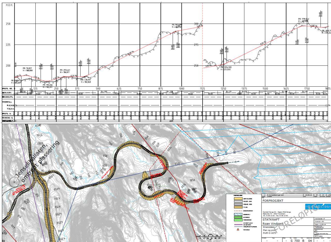
Figur 6: Eksempel på plan-/profiltegninger fra Roan vindkraftanlegg
